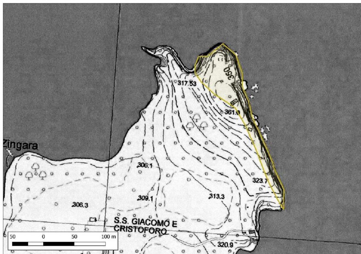
Ubicazione del geosito n. 68
