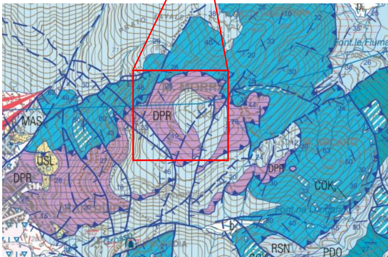
Stralcio geologico FOGLIO PALOMBARA SABINA 366 - 1:50.000
