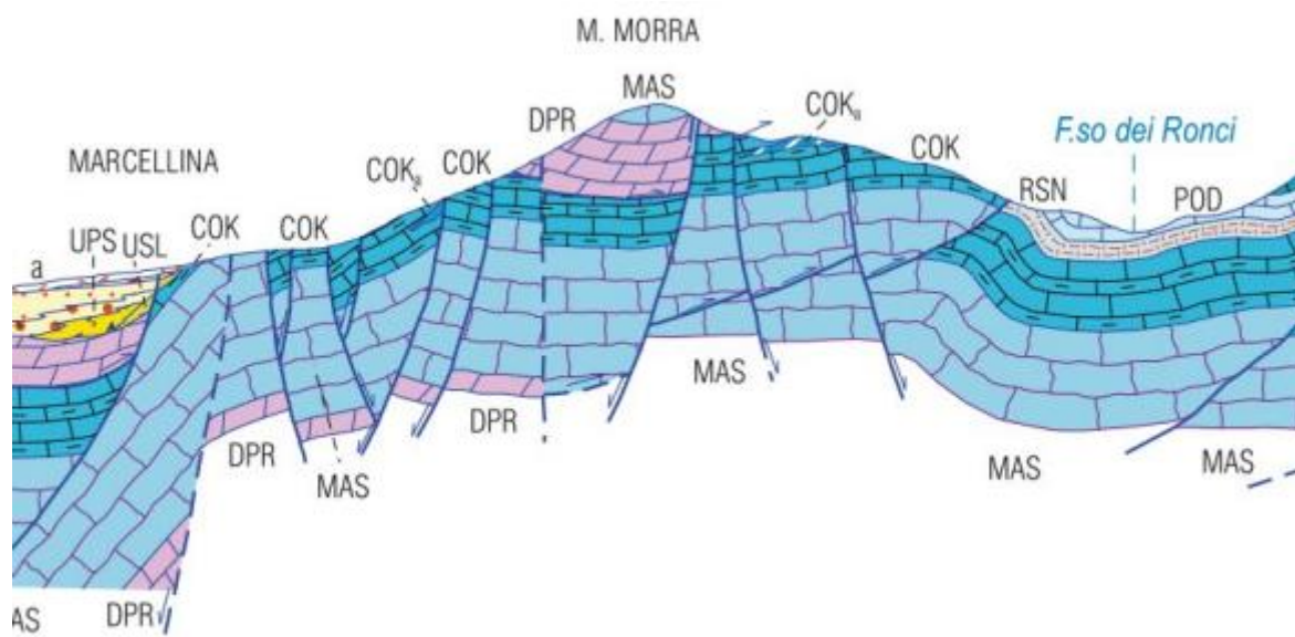
Sezione del Monte Morra
