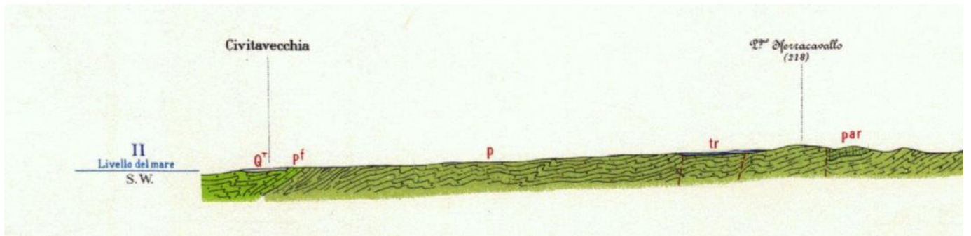
Sezione geologica
