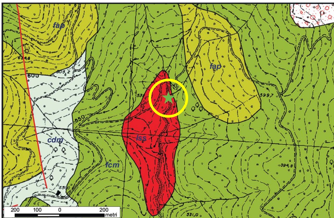
Stralcio Carta Geologica – Scala 1.25.000 – Regione lazio
