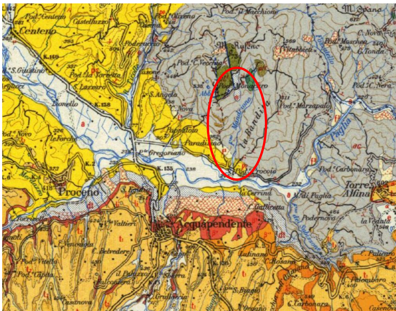
Stralcio carta Geologica al 100.000 – Foglio 129 – S.Fiora - In rosso area di studio
