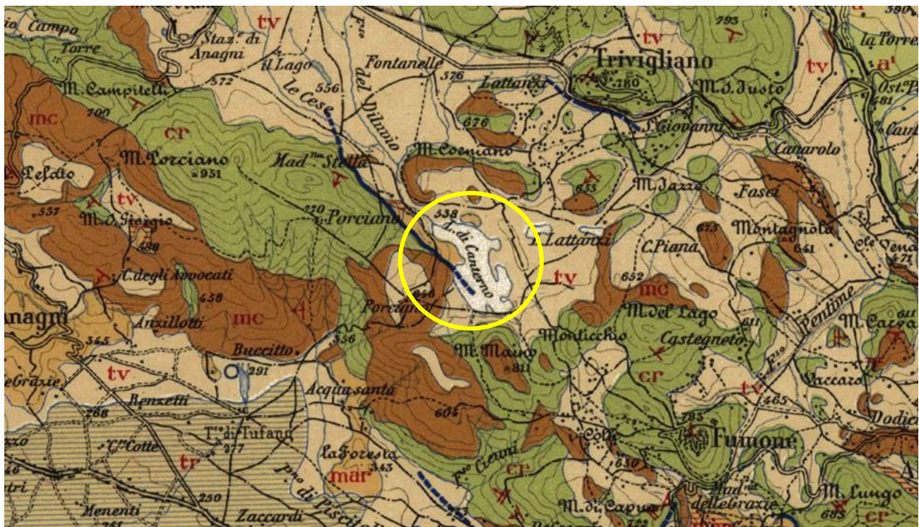
Stralcio carta geologica – Foglio ALATRI 151 – Scala 1:100.000
