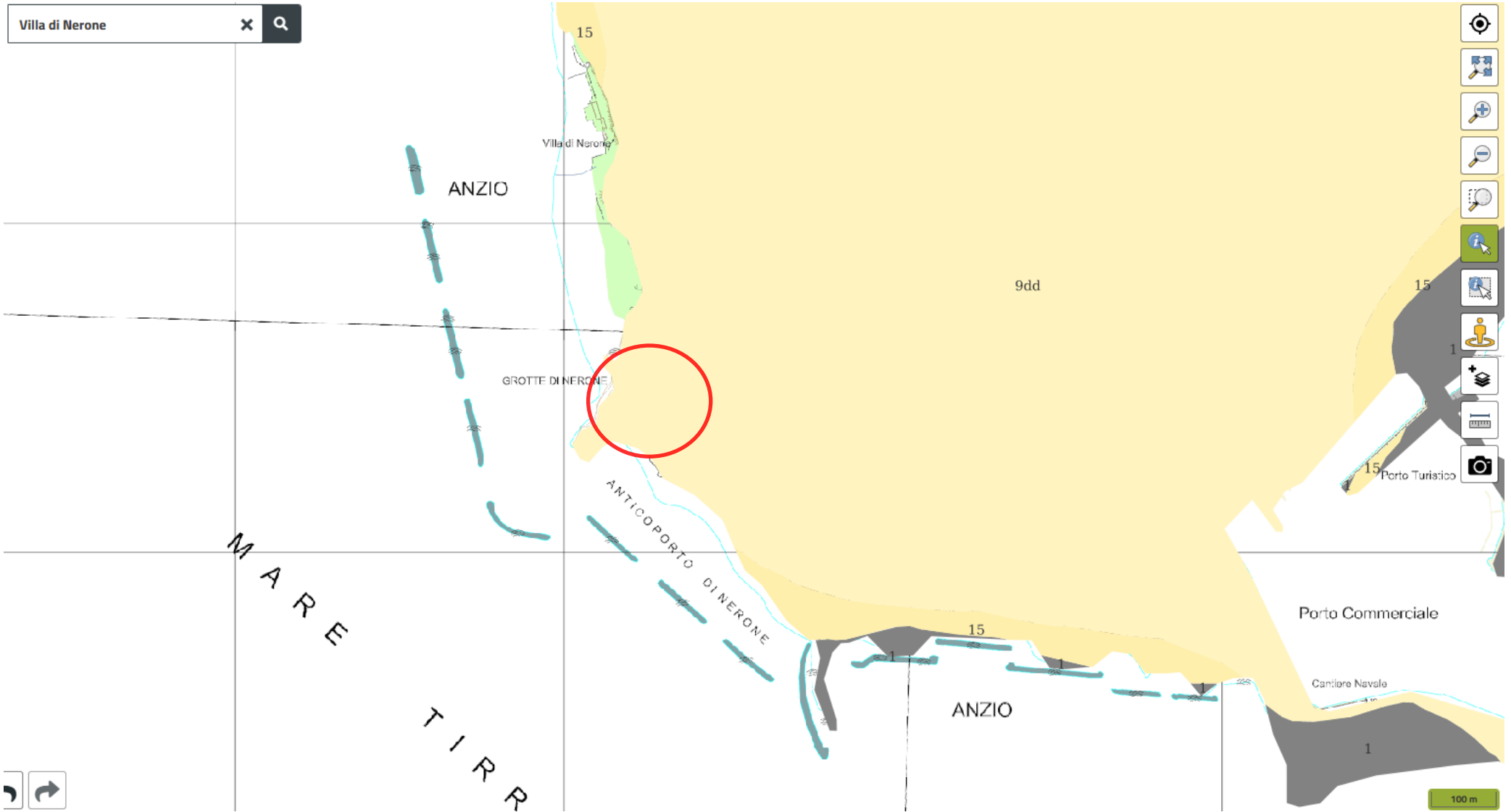
Stralcio Carta Geologica - Scala 1:25.000 - Regione Lazio
